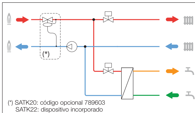
Diagrama hidráulico SATK204/SATK224
