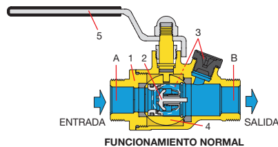
FUNCIONAMIENTO NORMAL
